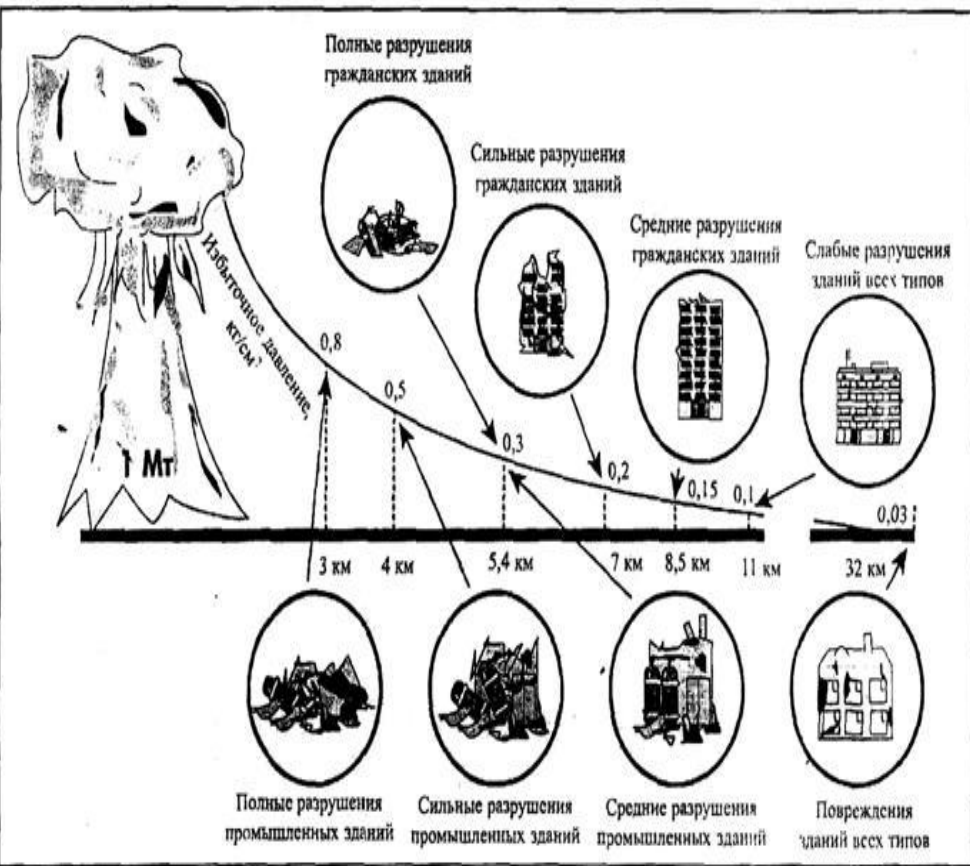
Рис. 28. Степень разрушения наземных зданий в зависимости от избыточного давления на фронте ударной волны, кг/см 2
