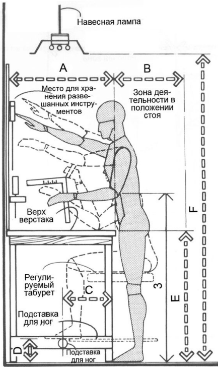
ВЫСОКИЙ ВЕРСТАК
