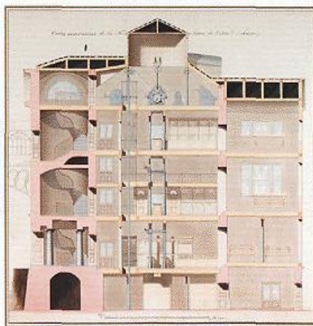
Чертеж мастерской по изготовлению хлопчатой пряжи. Разрез, 1830-е гг.
