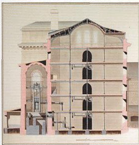
Чертеж льнопрядильной мастерской. Разрез, 1830-е гг.
