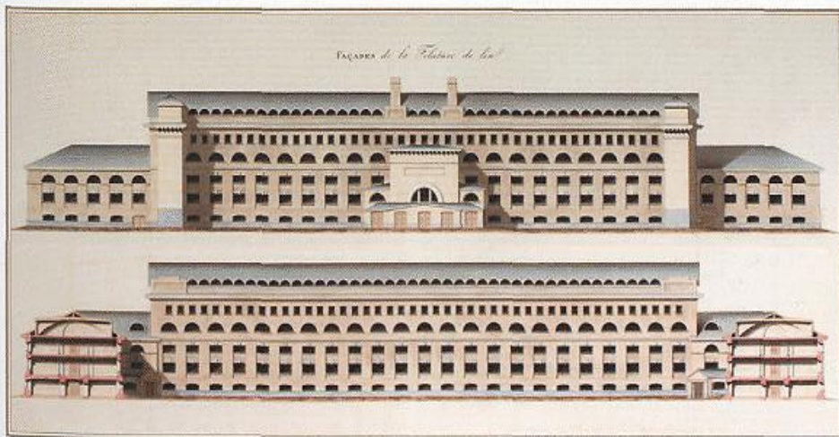
Чертеж здания льнопрядильной мастерской. 1830-е гг.
