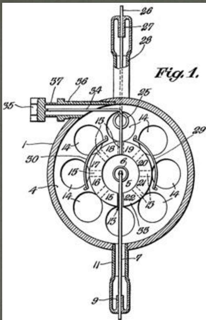
Магнетрон в поперечном сечении. Иллюстрация из патента № 2 408 235 от 24 сентября 1946 года. Уже получив 8 октября 1945 года патент на микроволновые печи, Перси Спенсер продолжал совершенствовать наиболее важную их деталь.
