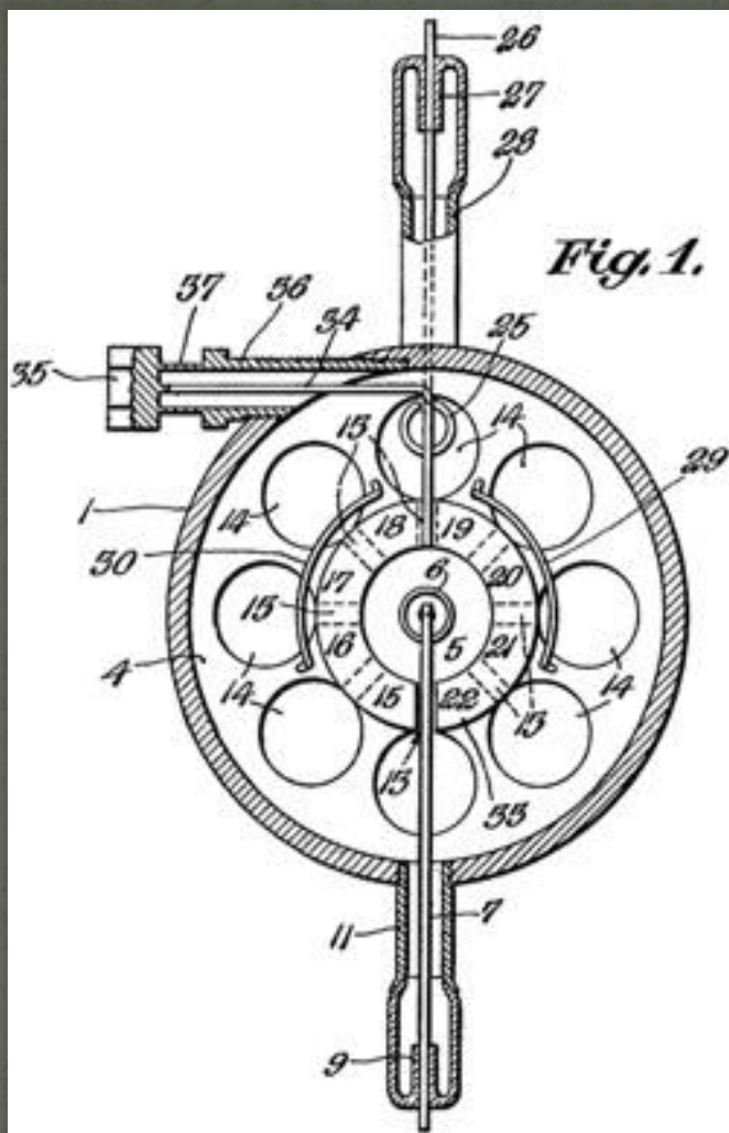
Магнетрон в поперечном сечении.
