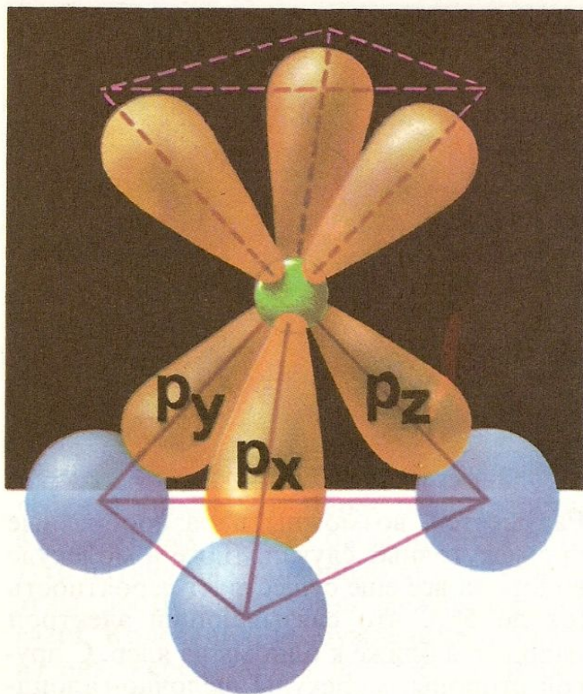
Рис. 155. Молекула аммиака \text{NH}_3 (расстояния между 2p -электронами сильно увеличены).
