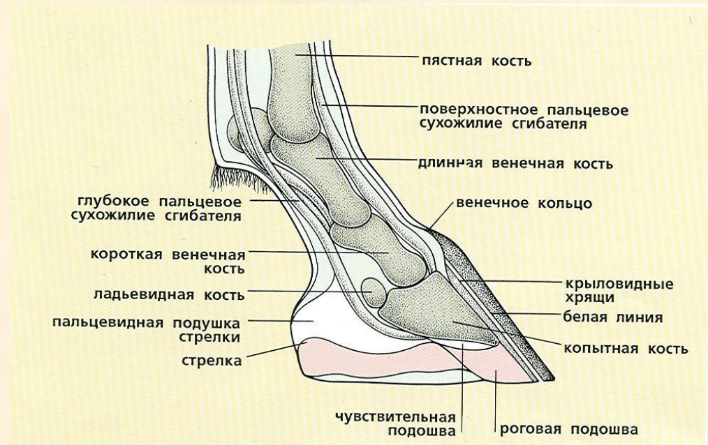
Рис.23 внутреннее строение копыта
