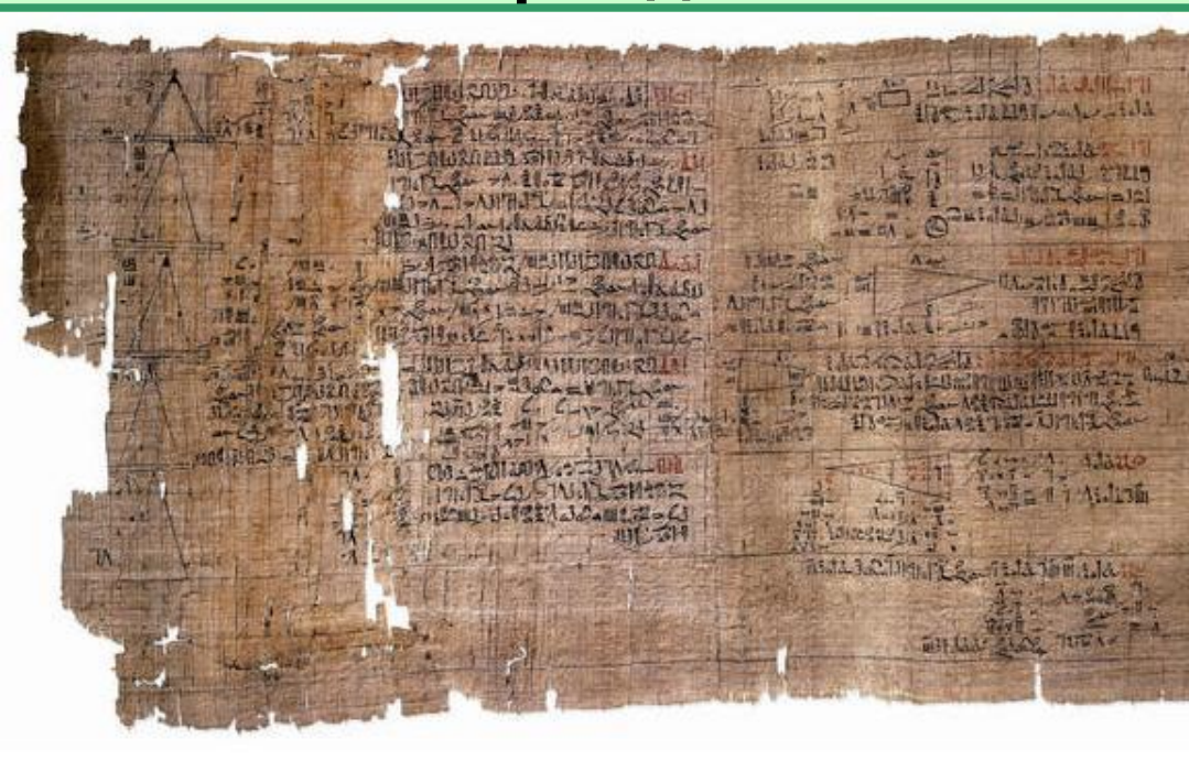
Часть папируса Ахмеса. Задачи с 49 по 55.
