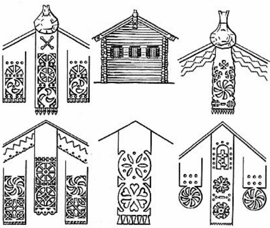
Рис. 79. СХЕМЫ СИМВОЛОВ СОЛНЦА И ЗЕМЛИ
