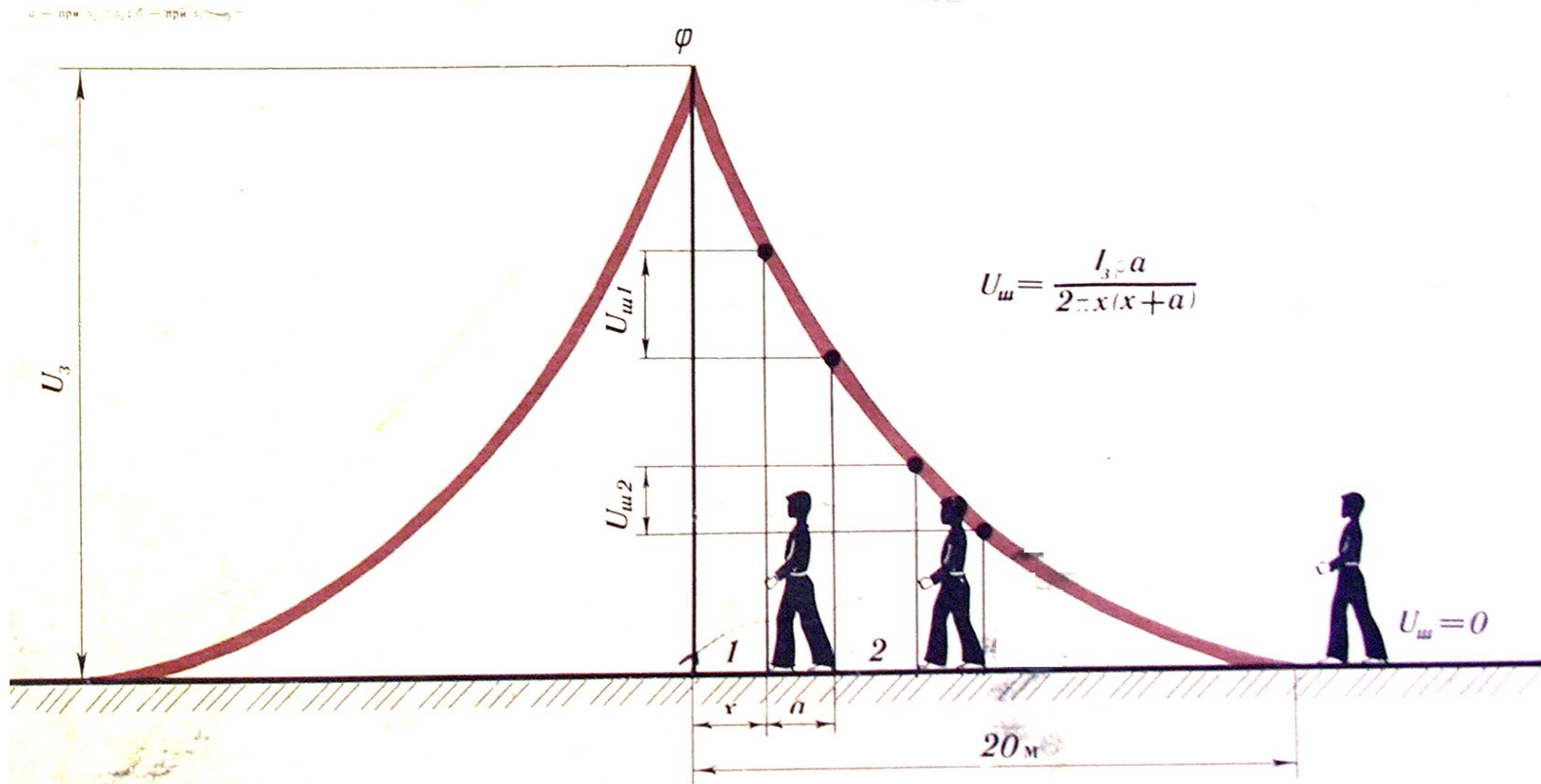
Рис. 3. Напряжение шага
