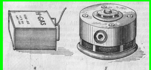
Рис. 5. Химические фугасы: а — фугас М1; б — фугас АВС-М23
