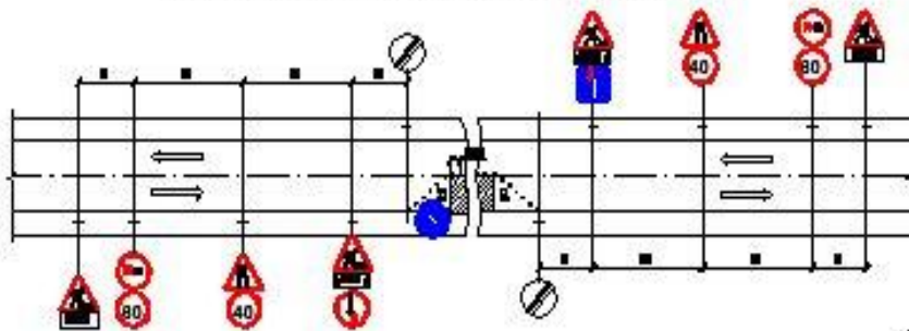
ОГРАЖДЕНИЕ МЕСТ РАБОТ, ВЫПОЛНЯЕМЫХ НА ПОЛОВИНЕ ШИРИНЫ ПРОЕЗЖЕЙ ЧАСТИ
