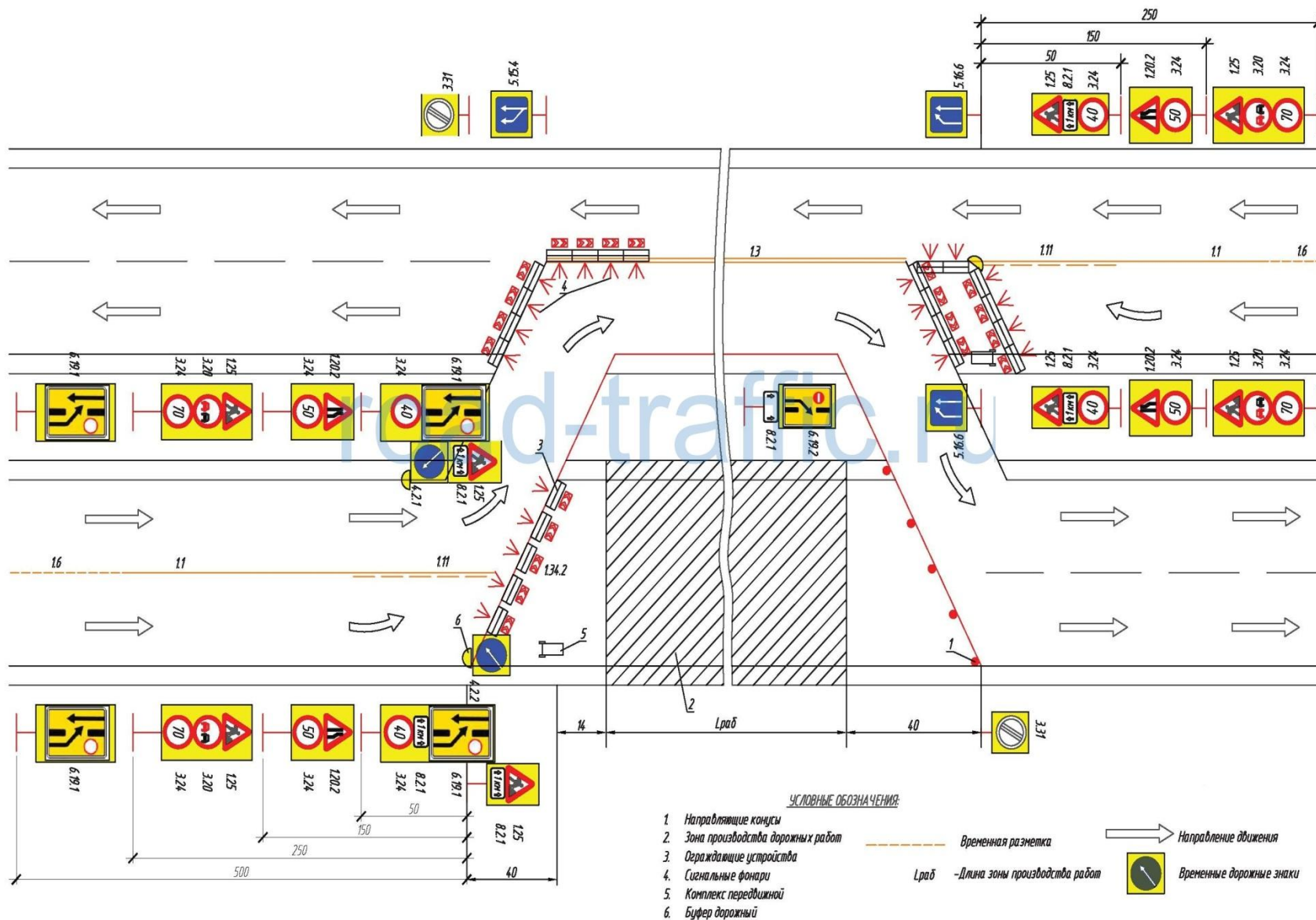
Схема организации движения и ограждение места производства дорожных работ, выполняемых на четырехполосных дорогах с закрытием движения по двум полосам
