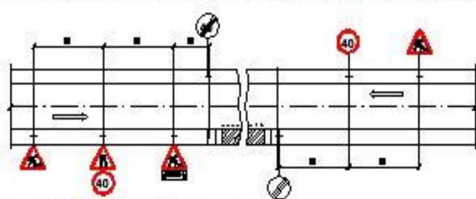
РАССТАНОВКА ЗНАКОВ В МЕСТАХ ПРИМЫКАНИЯ
