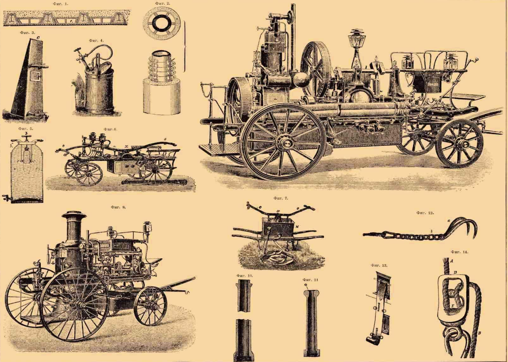
Фиг. 1—огнеупорное перекрытие. Фиг. 2—огнеупорная колонна. Фиг. 3—огнетушитель Шварца. Фиг. 4—ручной пожарный насос. Фиг. 5—звонилка Бабкока. Фиг. 6 и 7—ручные пожарные насосы. Фиг. 8—паровая пожарная труба. Фиг. 9—бензиновая пожарная труба. Фиг. 10—ствол брандспойта. Фиг. 11—наконечник брандспойта. Фиг. 12—ломовая веревка. Фиг. 13—спасательный крючок. Фиг. 14—тормозная веревка.
