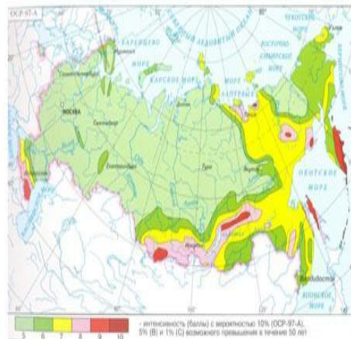
ОБЩЕЕ СЕЙСМИЧЕСКОЕ РАЙОНИРОВАНИЕ
