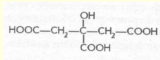
КИСЛОТИ
