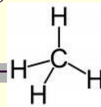
метан
