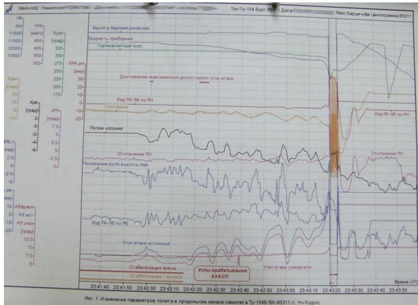
Рис. 1. Изменения параметров полета в продольном канале самолета Ту-154ВР-85311 (г. Уч-Кутуц).
