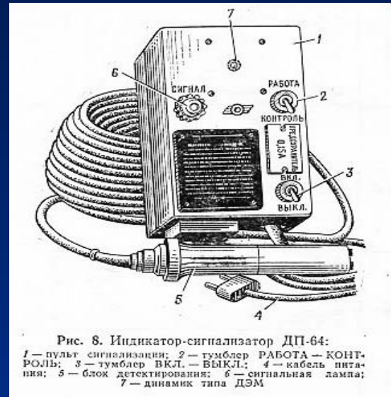
ИНДИКАТОР - СИГНАЛИЗАТОР ДП-64
