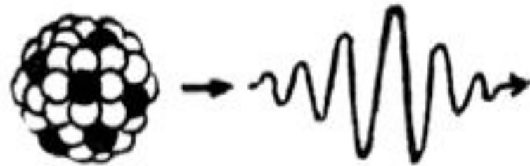
Гамма-квант
