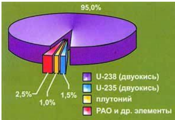
Состав ОЯТ
