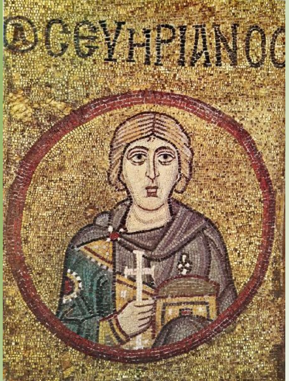
святий Севериан
