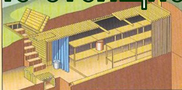
Отдельно стоящее противорадиационное укрытие из лесоматериалов
