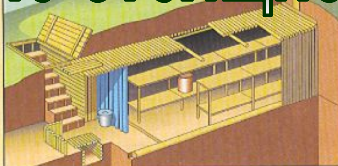
Отдельно стоящее противорадиационное укрытие из лесоматериалов
