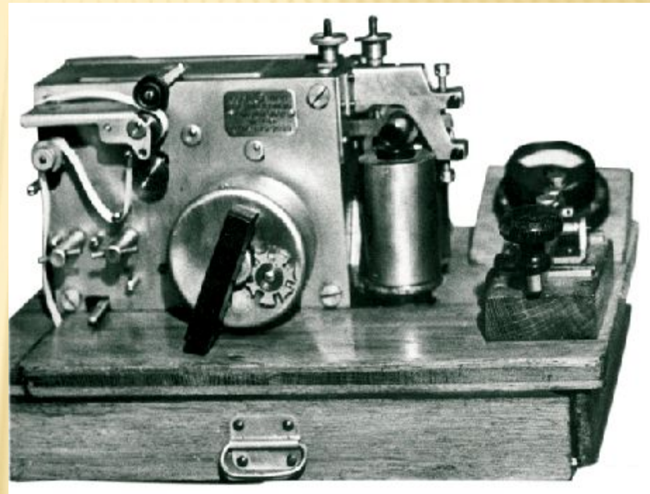
Телеграфный аппарат С.Морзе.
