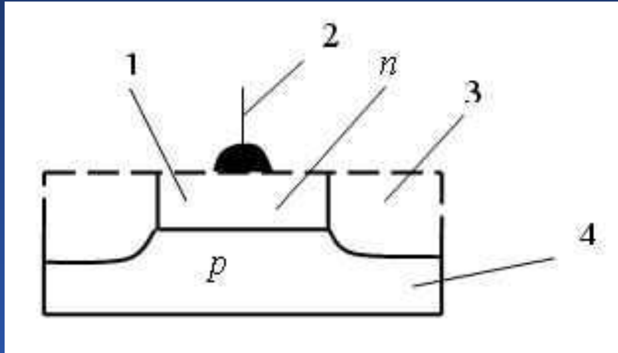
Устройство мезадиода
