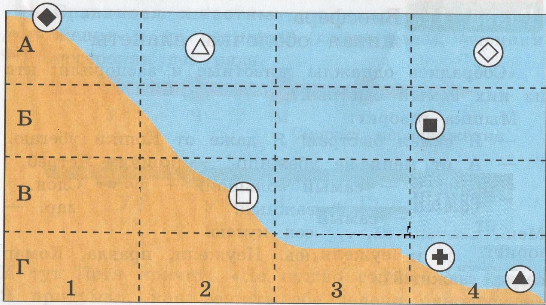
Профиль морского дна
