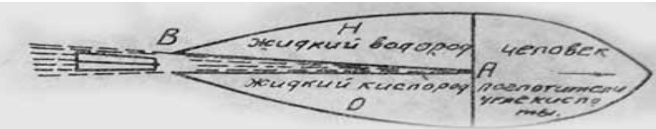
Ракета 1903 года.
