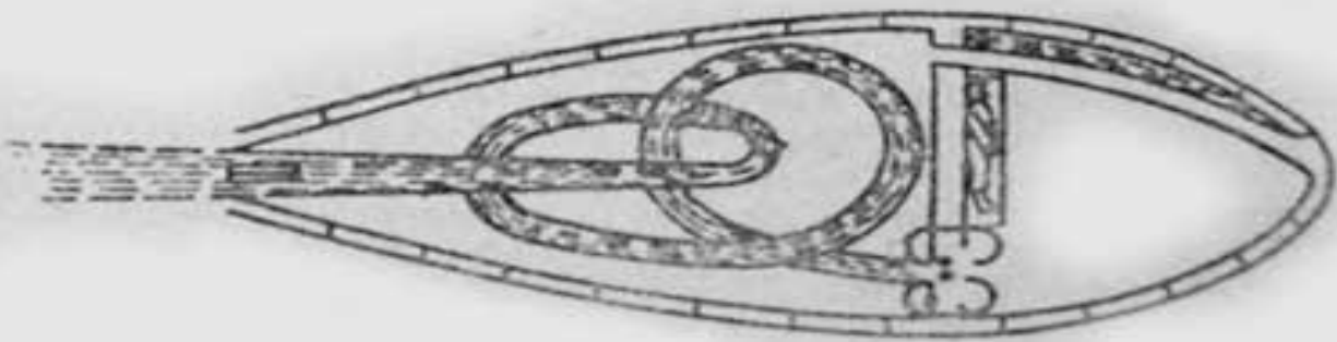
Ракета 1914 года.
