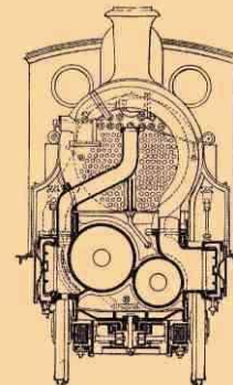
Черт. 6. Коммунальный паровоз Воределя (Worsdell).
