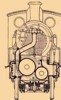
Черт. 6. Коммунальный паровоз Воределя (Worsdell).
