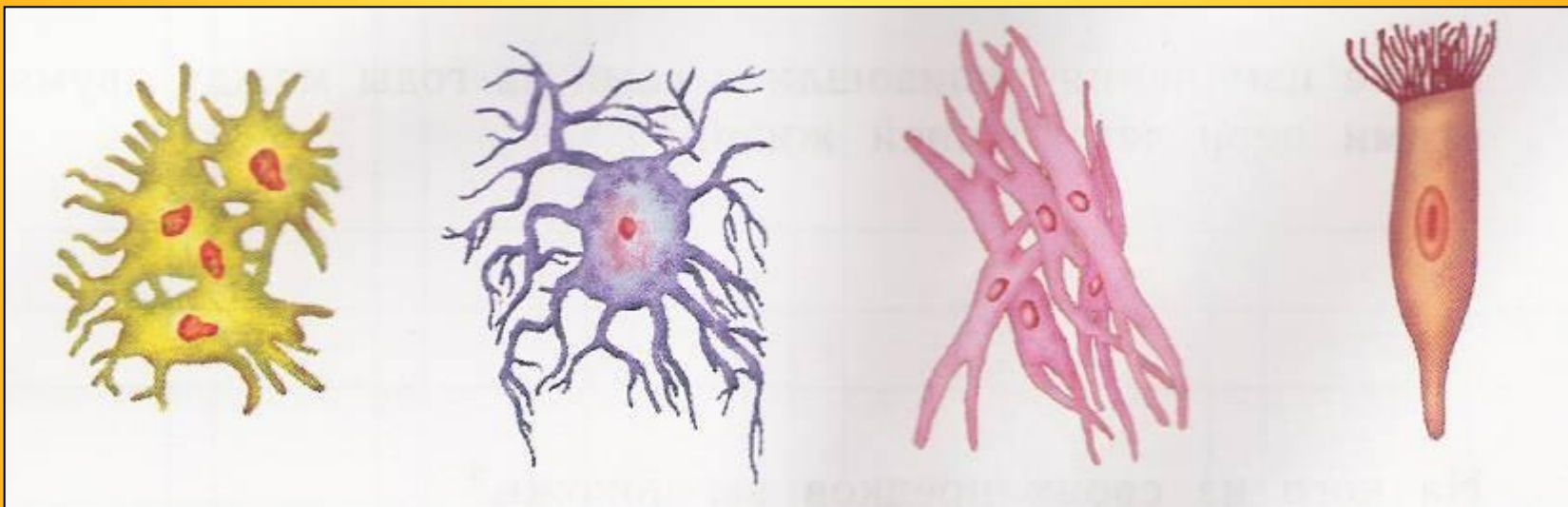
Клетка эпителия
