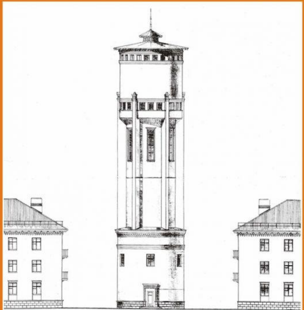
Один рабочих проектов Водонапорной башни, выполненных в марте 1953 года.
