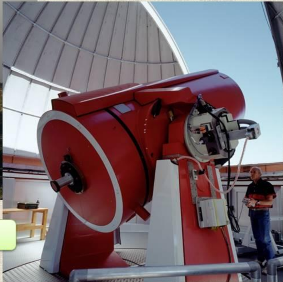
Телескоп
