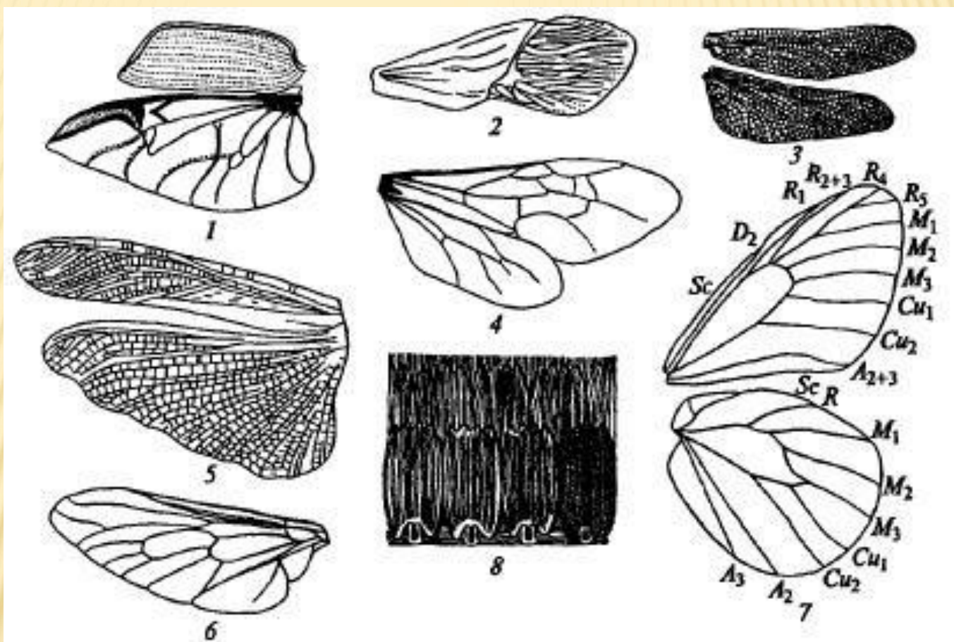
Рис. 1.4. Крылья насекомых:
