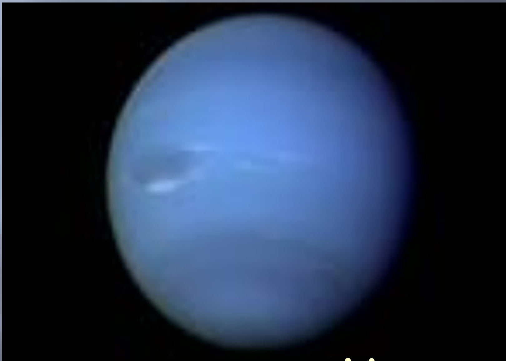
Нептун
