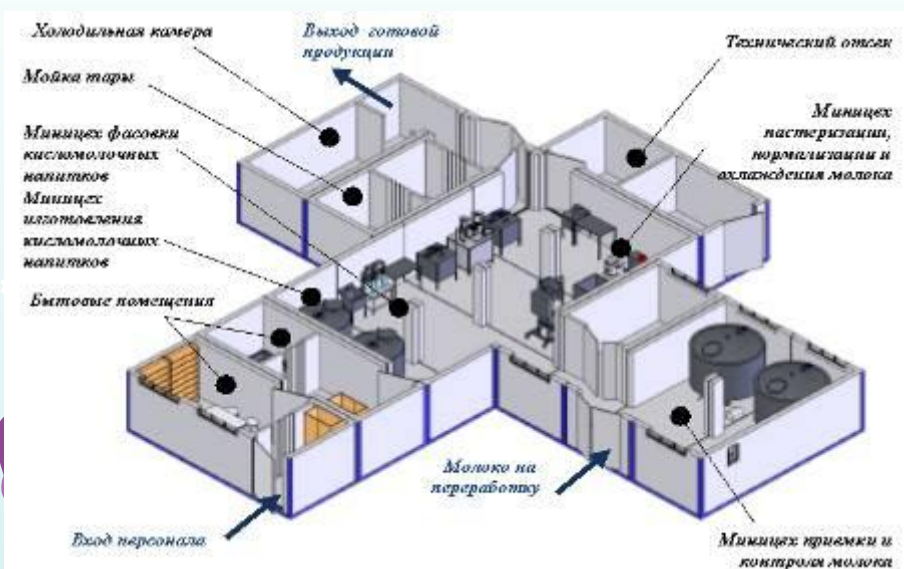
Схема маслозавода
