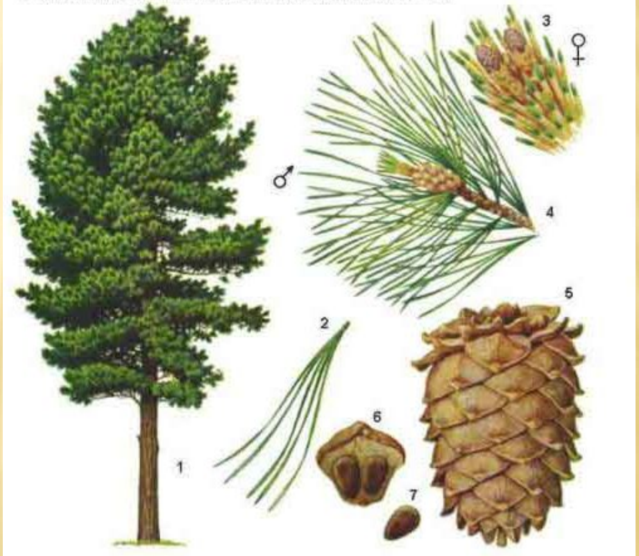
Кедровая сосна сибирская: 1 - общий вид дерева, 2 - укороченный побег с пятью хвоинками, 3 - верхушка удлиненного побега с женскими шишечками и развивающимися хвоинками, 4 - побег с мужскими колосками, 5 - зрелая шишка, 6 - одревесневшая семенная чешуя с двумя семенами, 7 - семя
