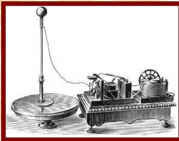
Радиоприемник А.С.Попова
