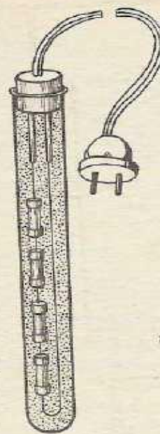
Аквариумный нагреватель из остеклованных сопротивлений.
