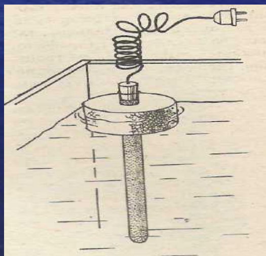
Аквариумный нагреватель на плавке из пенопласта.
