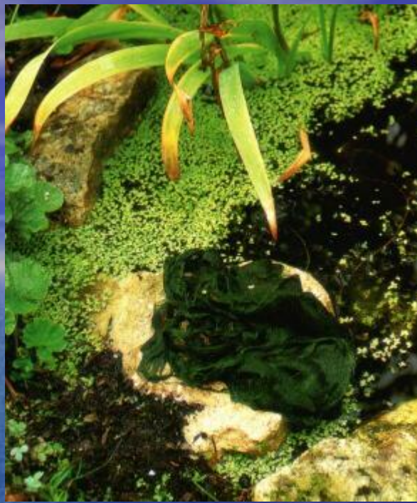
Водоросли спирогира
