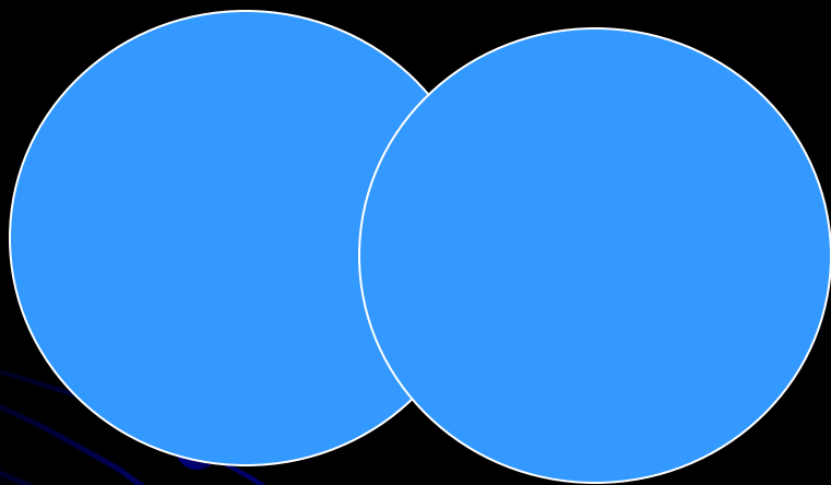
Молекула кислорода
