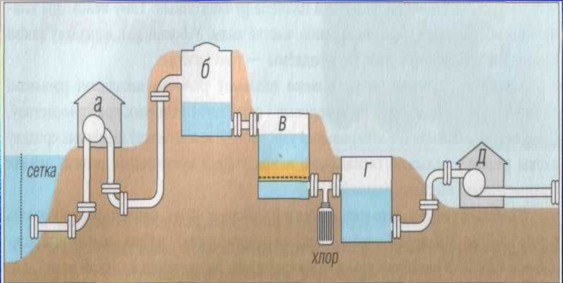
Мал. 118. Схема ачысткі пітной вады: а — помпа для падачы вады; б — адстойнік; в — пясчаны фільтр; г — зборнік чыстай вады; д — помпа для падачы вады спажыўцам
