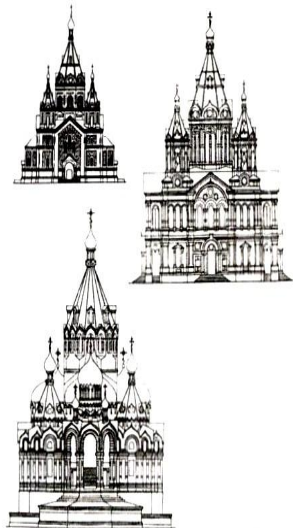
Рис. 4. Александро-Невский собор: вверху слева – фасад осуществленного собора 1883 года; справа – проект фасада собора, арх. Р. Килевейн, 1864; внизу – проект фасада открытой часовни с расширением, арх. Л. Даль, 1867. Чертеж автора
