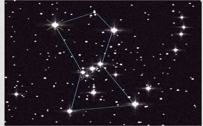
Созвездия
