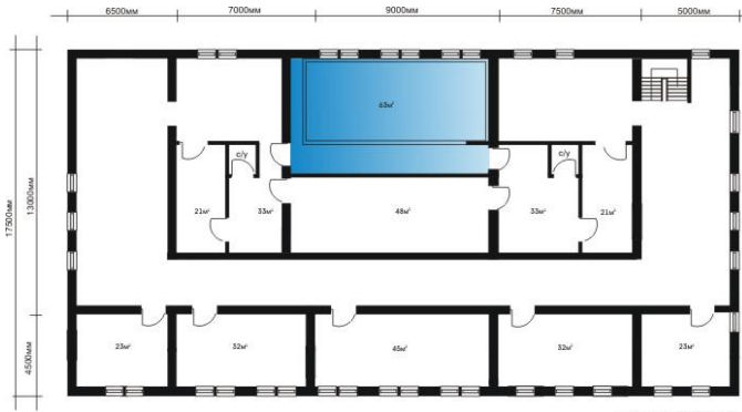
ПЛАН Золотая М 1:100
