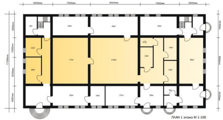
ПЛАН 1 этажа М 1:100
