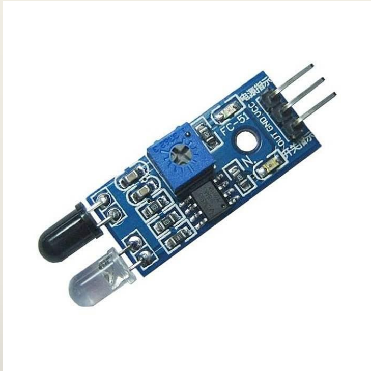
Инфракрасный датчик обнаружения препятствий.
