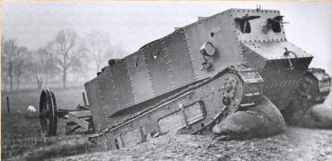
танк У.Свинтона
