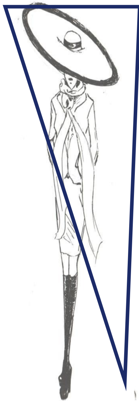
Треугольник
