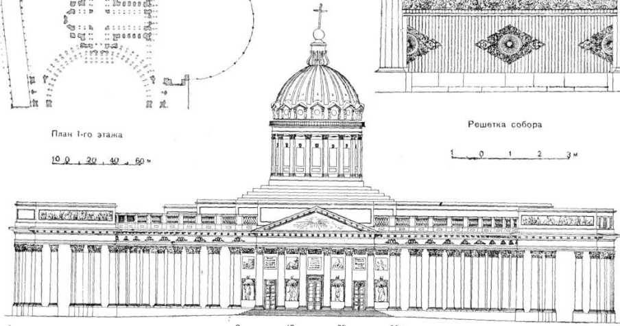
Северный фасад 0 10 20 30 м
