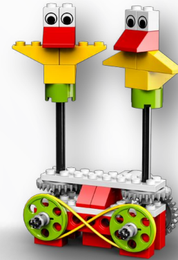
Ременная перекрёстная передача
