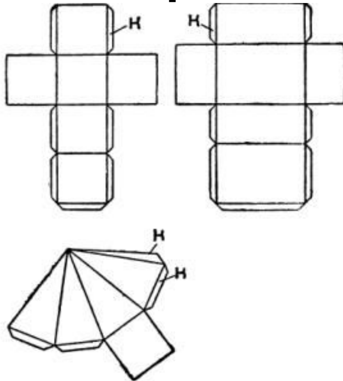
Рис. 119. Развёртки куба, параллелепипеда и пирамиды. H — клапаны, необходимые для склеивания геометрических тел.
