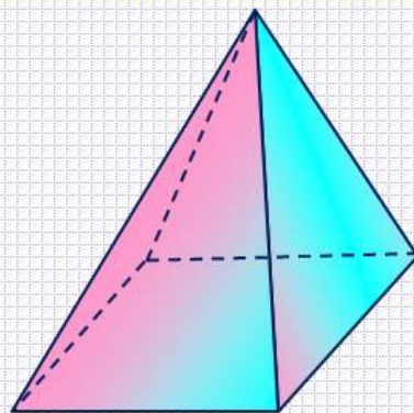
Четырехугольная пирамида
