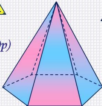
Шестиугольная пирамида
