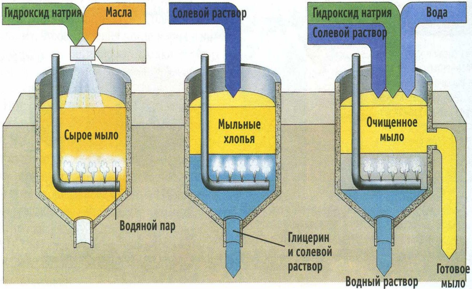
Промышленный способ производства мыла
