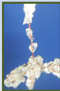
Выращивание кристаллов.
