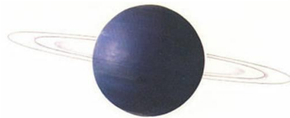
Нептун
