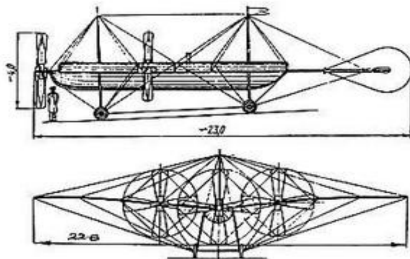
Первый в мире самолёт Можайского А.Ф. 1882 г.
